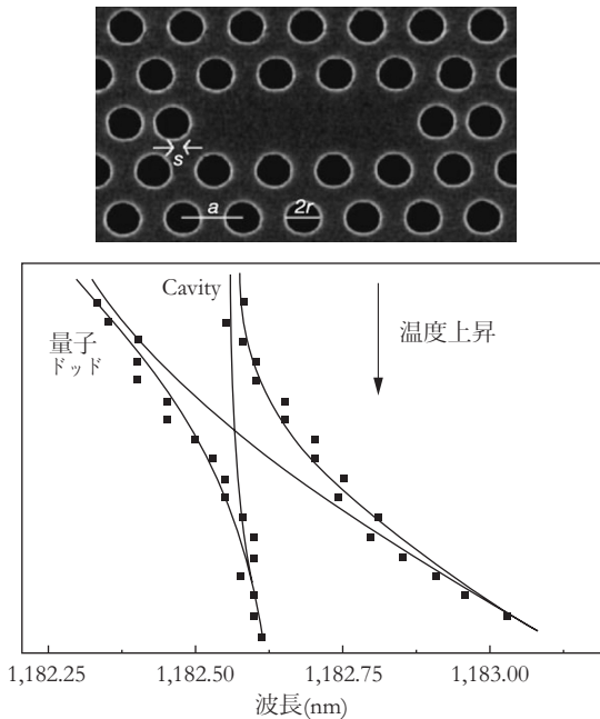
図 11 真空ラビ分裂の観測。(上)フォトニック結晶共振器の電子顕微鏡写真、(下)温度変化に伴う発光ピーク周波数の変化(出典: Nature , vol. 432, P. 200)
